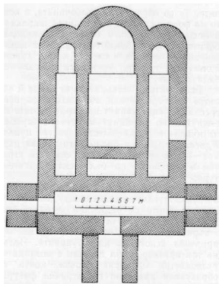
Обр. 1. Базиликата "Гебе клисе" в Преслав - план (по Н. Мавродинов).
